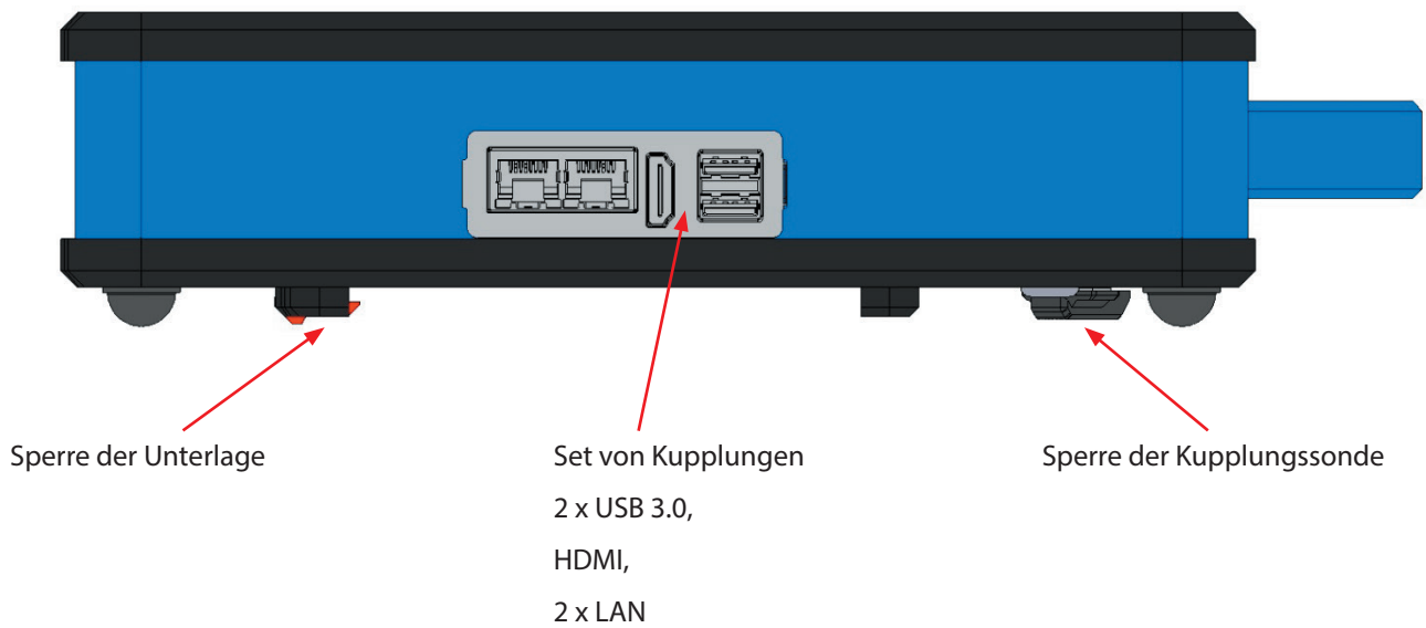
Abb. Gehäuseelemente. Ansicht von rechts.
